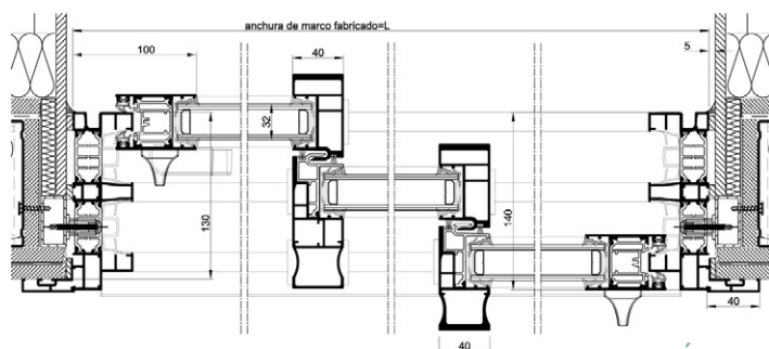
3 RAÍLES
